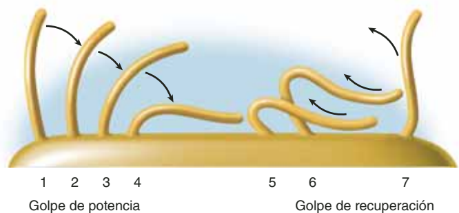
FIGURA 3.12 Acción ciliar. a) El cilio de un epitelio que mueve moco a lo largo de una capa superficial salina. b) Golpes de potencia y recuperación de un cilio individual.
